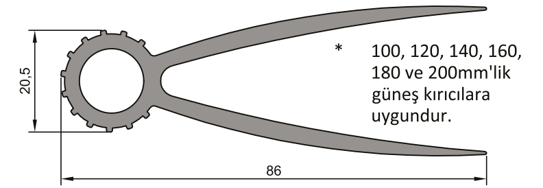
ER 9219 1,483 kg/m
