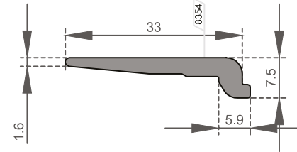
OM-5120 Cam Takoza / Glass Cleat Ağırlık / Weight 0,295 kg/m
