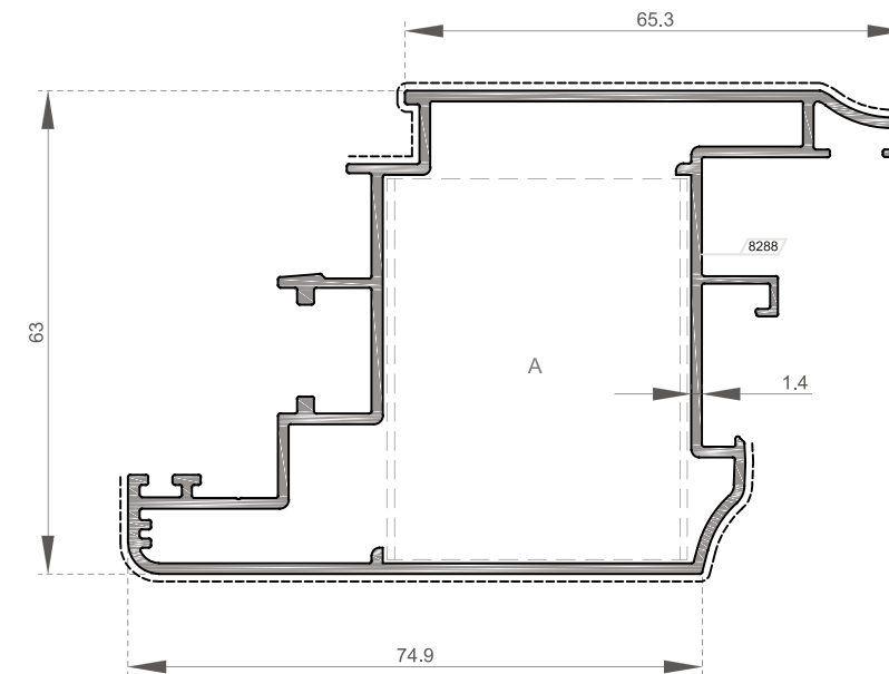
PL-3620 Kapı Kanadı Profili 65.3/ 74.9 / Door Sash Profile 65.3/ 74.9 Et Kalınlığı / Wall Thickness 1.4mm
