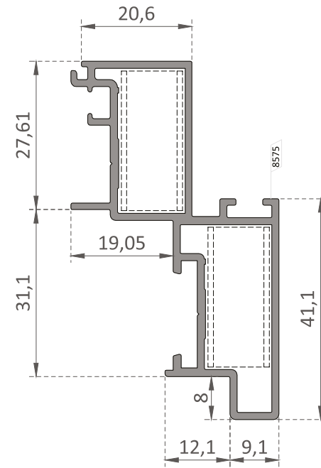
EL-1421 Kanat Profili / Sash Profile
