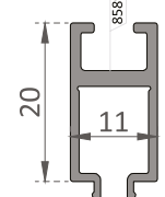
EL-2152 20 mm Yükseltme Profili / 20 mm Glazing Boost Profile
