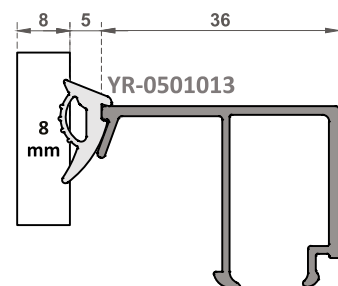
OM-6132 Cam Çıtası / Glazing Beads Ağırlık / Weight 0,367 kg/m
