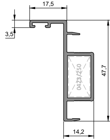
ER 9422 Çift Kanat Orta Adaptör Profili Double Sash Adapter Profile 0,491 kg/m
