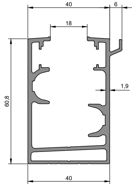
ER 9520 Kasa Profili Frame Profile 1,374 kg/m
