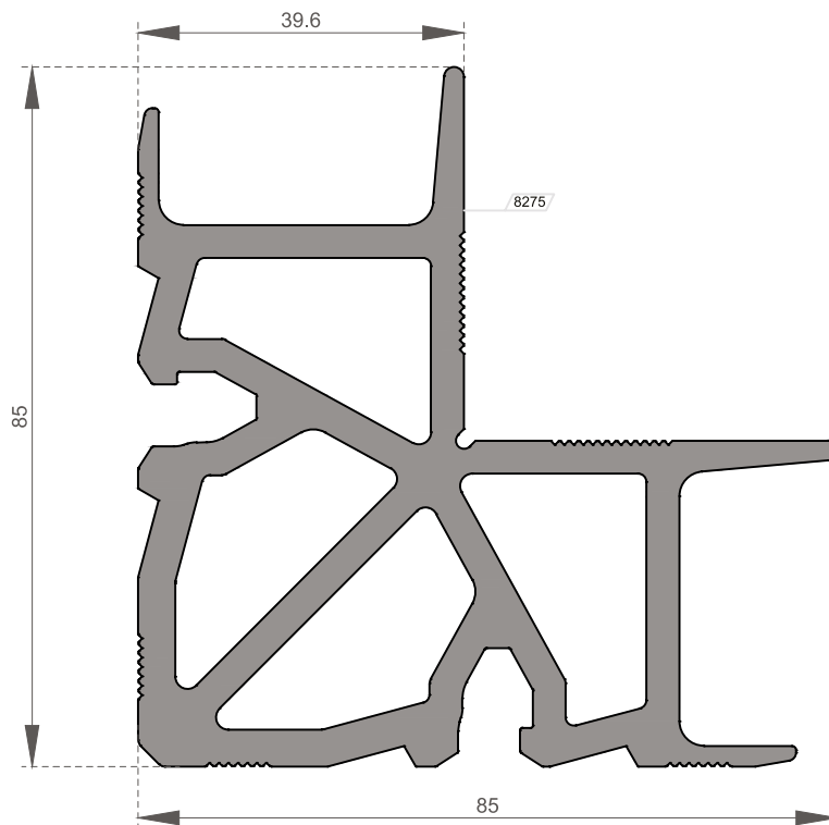
OM-5114 Köşe Takoz Profili / Corner Cleat Profile Ağırlık / Weight 4,724 kg/m
