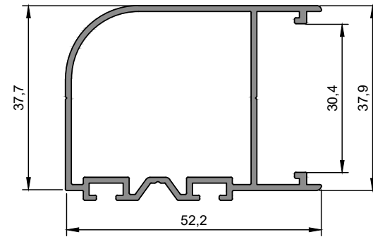
ER 9519 90° Köşe Dönüş Profili 90° Corner Profile 0,650 kg/m
