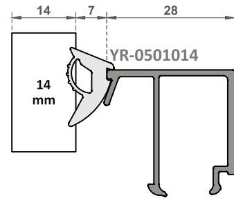
OM-6123 Cam Çıtası / Glazing Beads Ağırlık / Weight 0,335 kg/m
