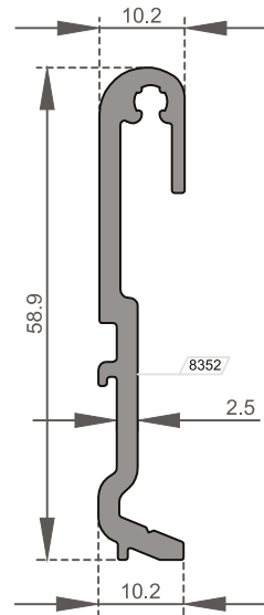
OM-5211 T Bağlantı Profili / T Connection Profile Ağırlık / Weight 0,592 kg/m
