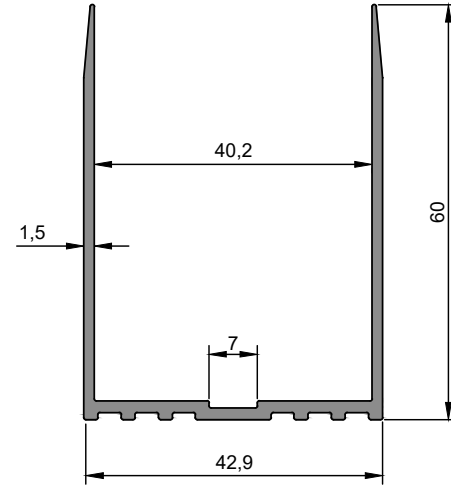
ER 9518 Kasa Boşluk Kapatma Profili Frame Cover Profile 0,683 kg/m
