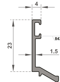
OM-5340 Katlanır Kapı Üst Kapama Profili / Closing Profile for Folding Door
