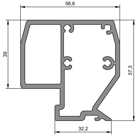
ER 9253 U Bağlantı Profili U Connection Profile 1,827 kg/m
