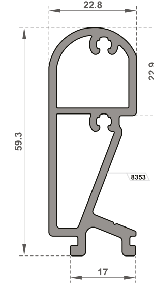
OM-5212 U Bağlantı Profili / U Connection Profile
