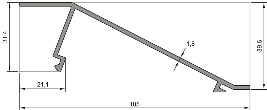
ER 9241 0,762 kg/m
