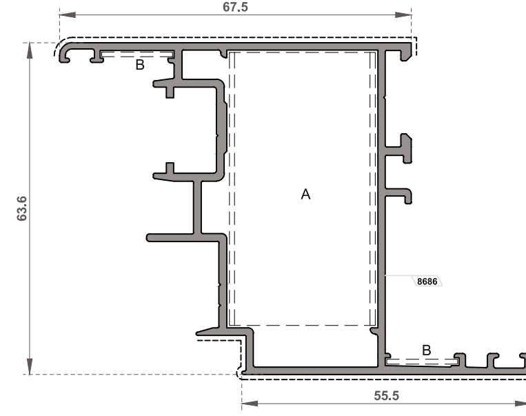
FI-3222 Kanat Profili 67.5/55.5 / Sash Profile 67.5/55.5 Et Kalınlığı / Wall Thickness 1.5mm
