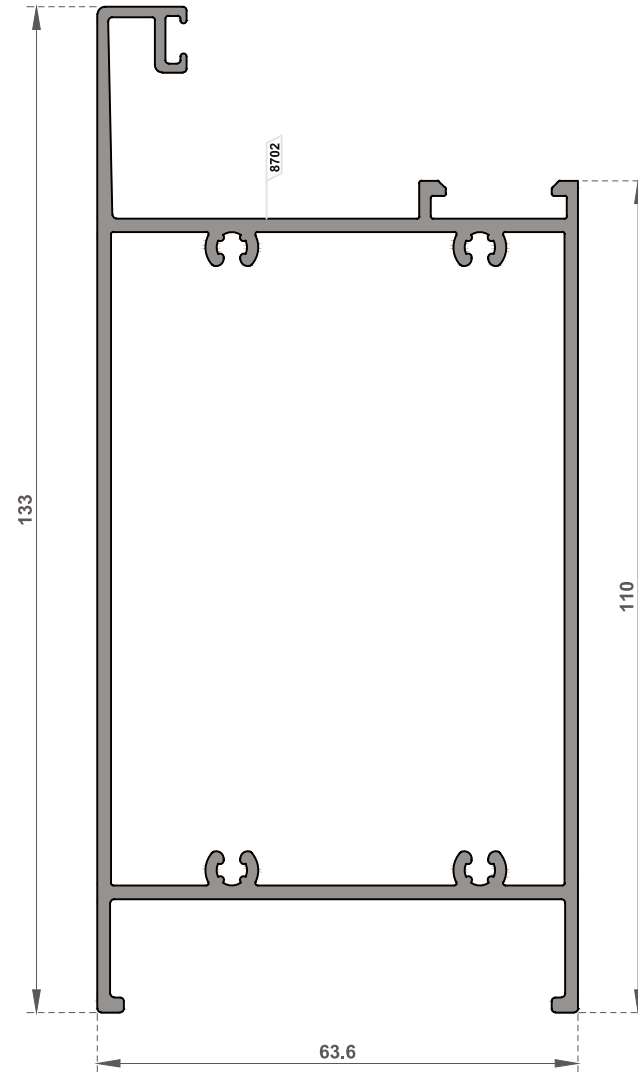
FI-4330 Dışa Açılır Kapı İçin Etek Profili / Bottom Plate Profile for Outward Opening Door
