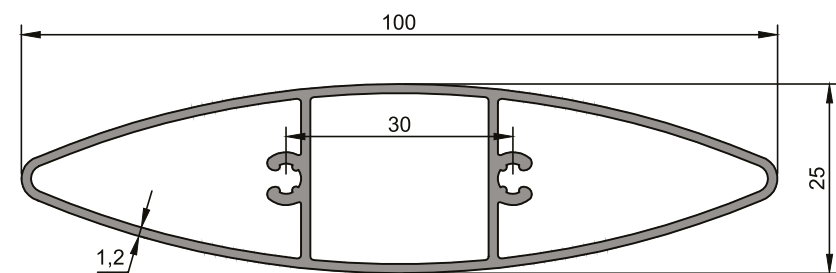
ER 9211 0,905 kg/m
