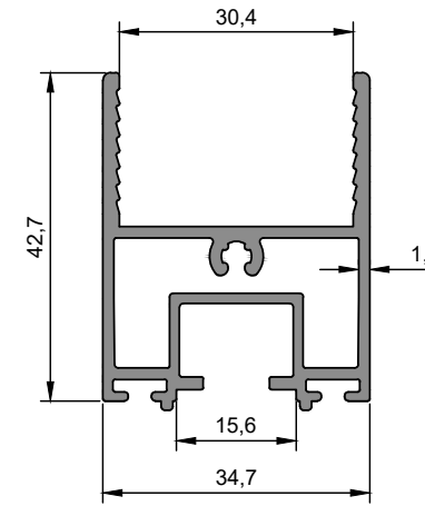
ER 9803 30 mm Isıcamlı Kanat Profili Sash Profile for 30 mm Glazing 0,846 kg/m
