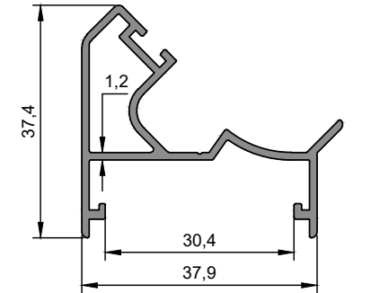
ER 9521 135° Köşe Dönüş Profili 135° Corner Profile 0,462 kg/m
