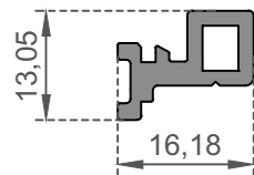
ER 9401 Kitleme Profili Interlocking Profile Ağırlık / Weight 0,233 kg/m
