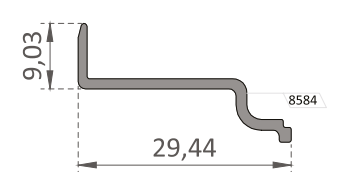
EL-2144 Cam Taşıyıcı Profili / Glass Support Profile
