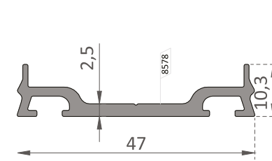
EL-1510 Baskı Profili / Pressure Profile
