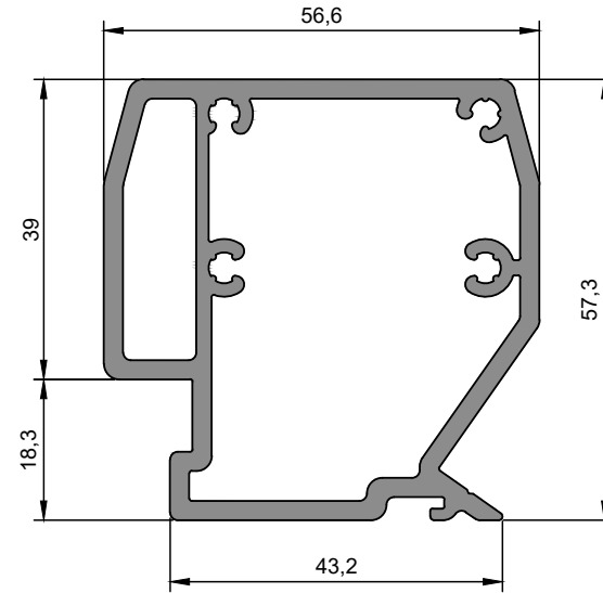
ER 9254 U Bağlantı Profili U Connection Profile 1,827 kg/m
