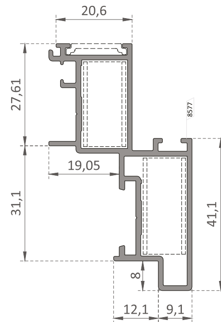
EL-1422 Kanat Profili / Sash Profile
