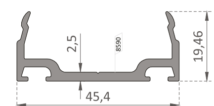
EL-1520 Baskı Kapak Profili / Glass Spacer Profile
