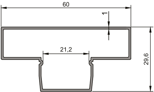
ER 8266 0,474 kg/m
