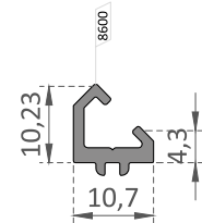
EL-2410 Açılı Kapak Profili / Angular Cover Profile
