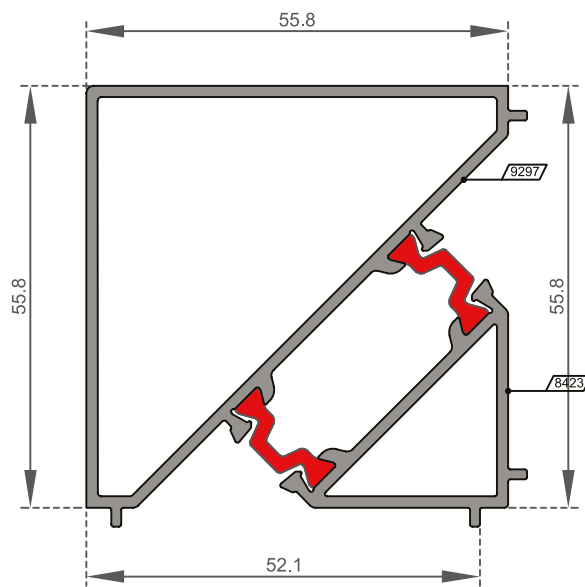
OM-5811 90° Köşe Adaptör Profili / 90° Corner Adapter Profile Ağırlık / Weight 1,398 kg/m
