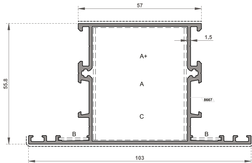
FI-2123 Orta Kayıt Profili 57/103 / Mullion Profile 57/103 Et Kalınlığı / Wall Thickness 1.5mm
