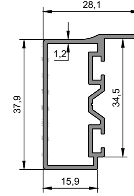
ER 9522 Yan Kasa Profili Side Frame Profile 0,463 kg/m
