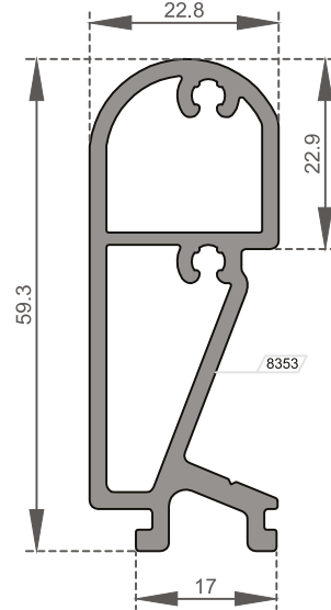
OM-5212 U Bağlantı Profili / U Connection Profile Ağırlık / Weight 1,021 kg/m
