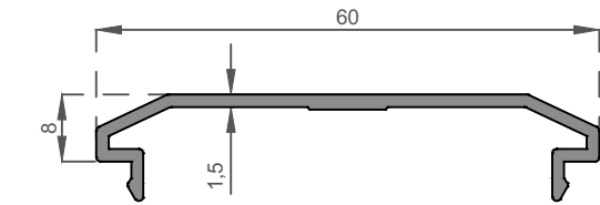
ER 9104 0,348 kg/m Çarpma Kapı Adaptör Profili Impact Door Adapter Profile
