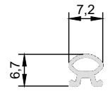
YR-0503001 SCHELEGEN Fitil SCHELEGEN Gasket
