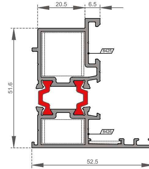
FS-5530 Dışa Açılır Adaptör Profili / Adapter Profile for Outward Opening Ağırlık / Weight 1,120 kg/m
