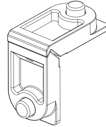
YR-0803006 KANAT: Monticelli Köşe Takozu 0423/250 (L:19, H:10.6)
