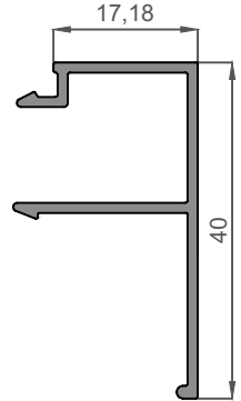
ER 8092 Cam Çıtası Profili Glazing Bead Profile Ağırlık / Weight 0,285 kg/m
