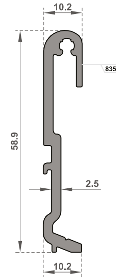
OM-5211 T Bağlantı Profili / T Connection Profile
