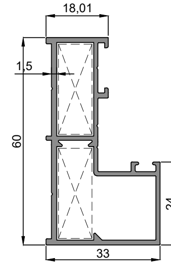
ER 9245 Kasa Profili Frame Profile 0,772 kg/m
