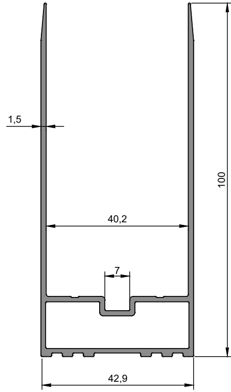
ER 9517 Kasa Boşluk Kapatma Profili Frame Cover Profile 1,145 kg/m
