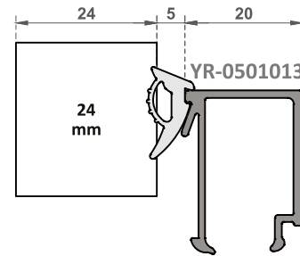
OM-6121 Cam Çıtası / Glazing Beads Ağırlık / Weight 0,302 kg/m
