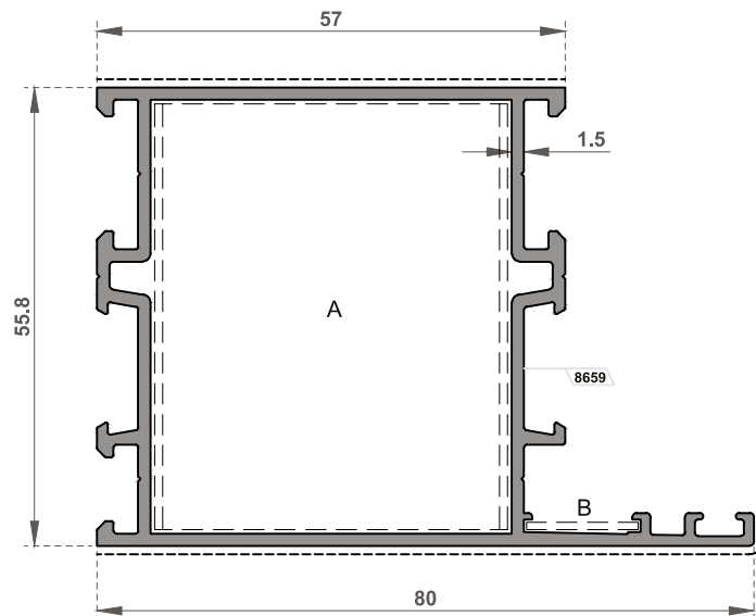
FI-1123 Kasa Profili 57/80 / Frame Profile 57/80 Et Kalınlığı / Wall Thickness 1.5mm
