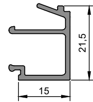
ER 9252 Cam Çıtası Profili Glazing Bead Profile 0,235 kg/m
