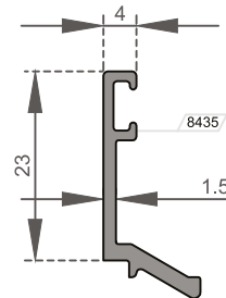
OM-5340 Katlanır Kapı Üst Kapama Profili / Closing Profile for Folding Door Ağırlık / Weight 0,176 kg/m
