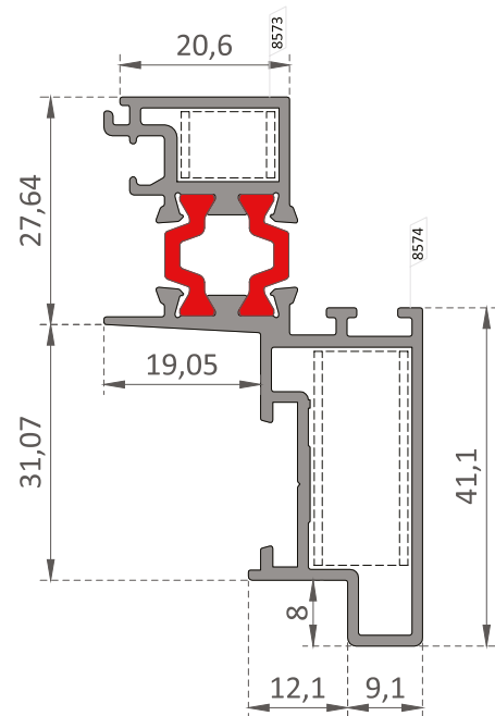
EL-1410 Kanat Profili / Sash Profile
