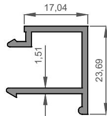
ER 3727 Tek Cam Çıtası Profili Glazing Bead Profile Ağırlık / Weight 0,285 kg/m
