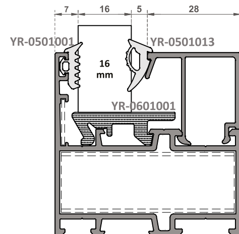
OM-6123 Cam Çıtası / Glazing Beads Ağırlık / Weight 0,335 kg/m
