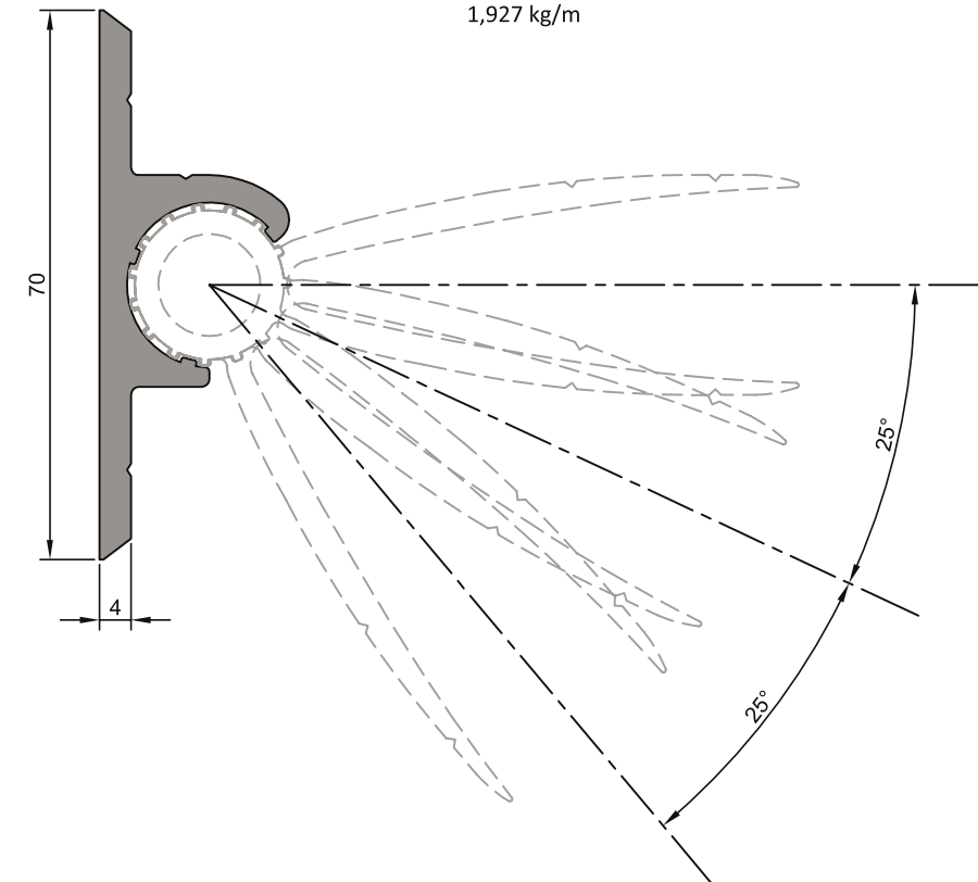
ER 9300 1,927 kg/m
