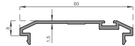
ER 3724 0,375 kg/m Çarpma Kapı Adaptör Profili Impact Door Adapter Profile
