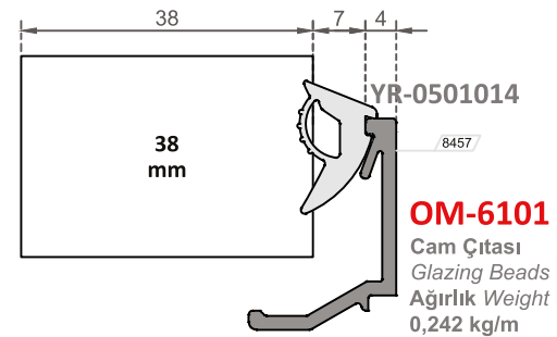
OM-6101 Cam Çıtası Glazing Beads Ağırlık / Weight 0,242 kg/m
