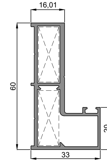
ER 9246 Cam Kapı Kasa Profili Frame Profile 0,855 kg/m
