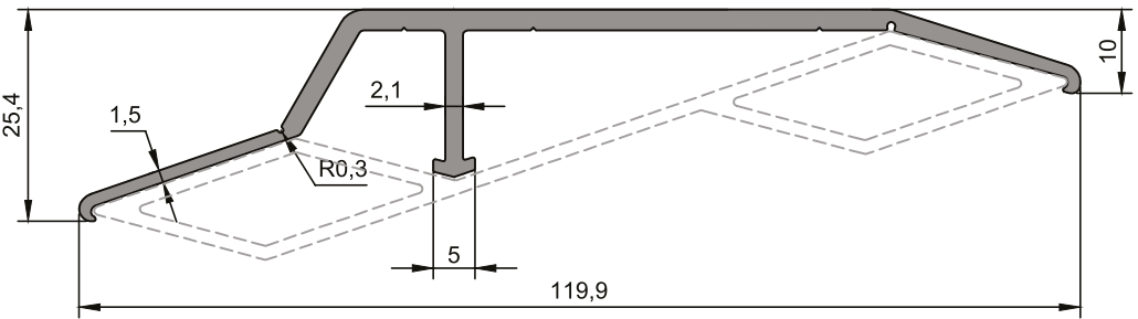
ER 8255 0,885 kg/m
