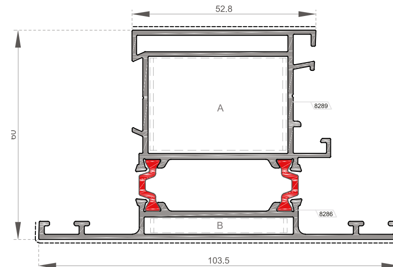
PS-1425 Geniş T Kasa Profili 52.8 / 103.5 / Wide T Frame Profile 52.8/ 103.5 Et Kalınlığı / Wall Thickness 1.5mm
