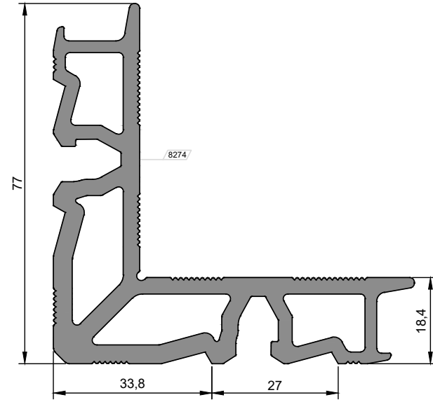
OM-5111 Köşe Takozu / Corner Cleat 3,061 kg/m
