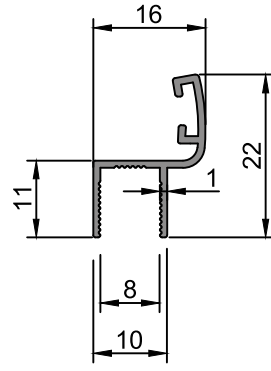
ER 6465 0,139 kg/m
