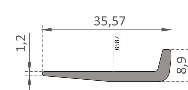
EL-2141 Cam Taşıyıcı Profili / Glass Support Profile
