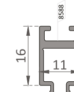
EL-2151 16 mm Yükseltme Profili / 16 mm Glazing Boost Profile
