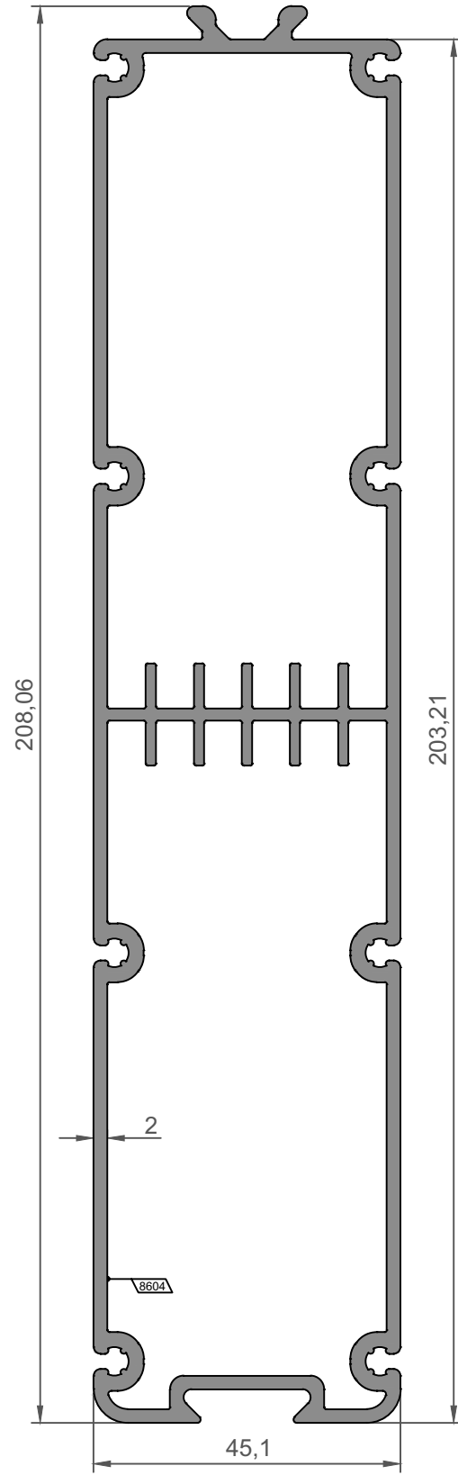
EL-2220 Dilatasyon Profili Dilatation Profile Ağırlık / Weight 3,742 kg/m
