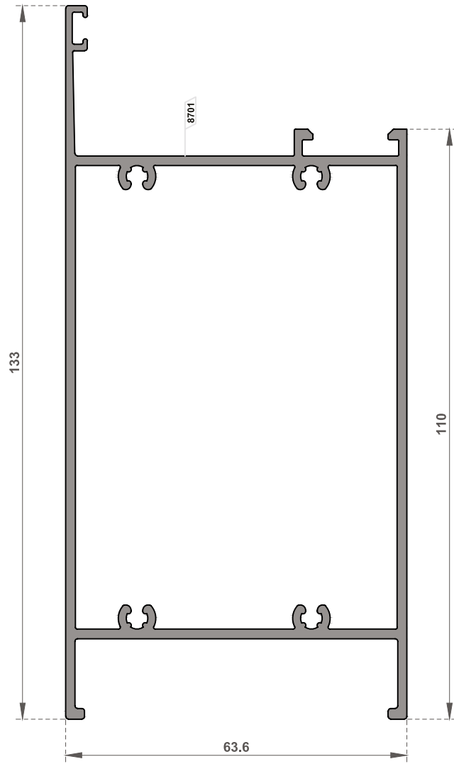
FI-4230 İçe Açılır Kapı İçin Etek Profili / Bottom Plate Profile for Inward Opening Door
