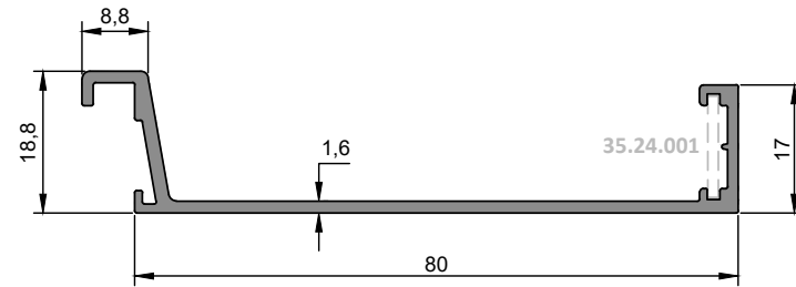
ER 9423 Adaptör Profili / Adapter Profile 0,569 kg/m
