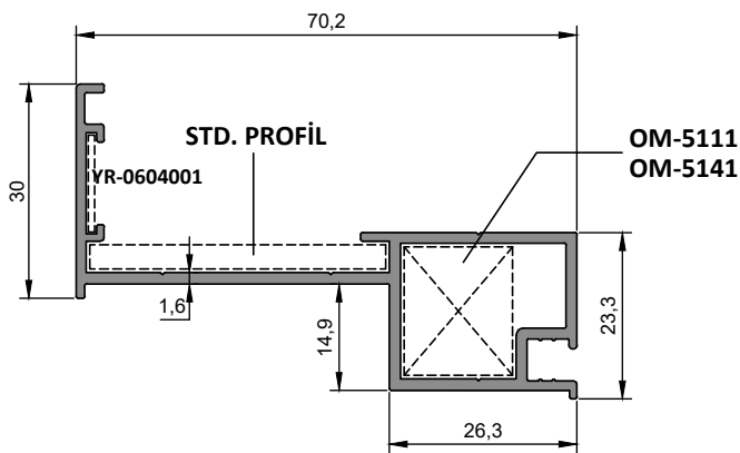
ER 9235 0,748 kg/m
