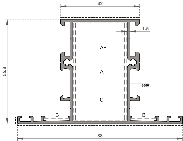
FI-2122 Orta Kayıt Profili 42/88 / Mullion Profile 42/88 Et Kalınlığı / Wall Thickness 1.5mm
