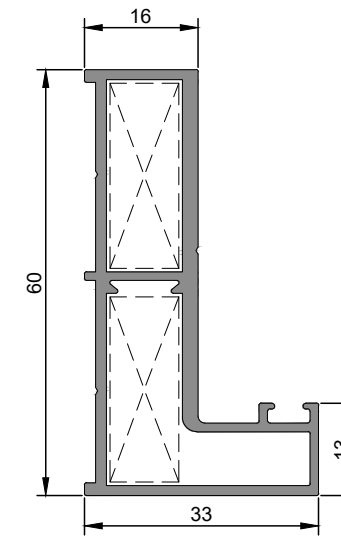
ER 9248 Ahşap Kapı Kasa Profili Frame Profile 0,867 kg/m
