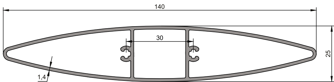
ER 9213 1,338 kg/m
