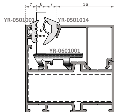
OM-6132 Cam Çıtası / Glazing Beads Ağırlık / Weight 0,367 kg/m
