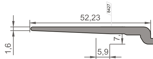
FT-5120 Cam Takoza / Glass Cleat Ağırlık / Weight 0,412 kg/m
