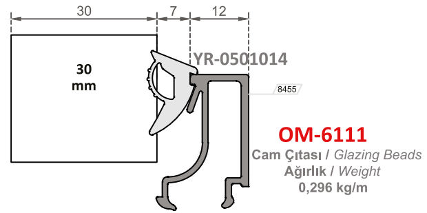
OM-6111 Cam Çıtası / Glazing Beads Ağırlık / Weight 0,296 kg/m
