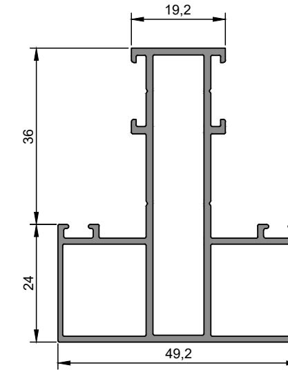
ER 9249 Orta Kayıt Profili Mullion Profile 0,978 kg/m
