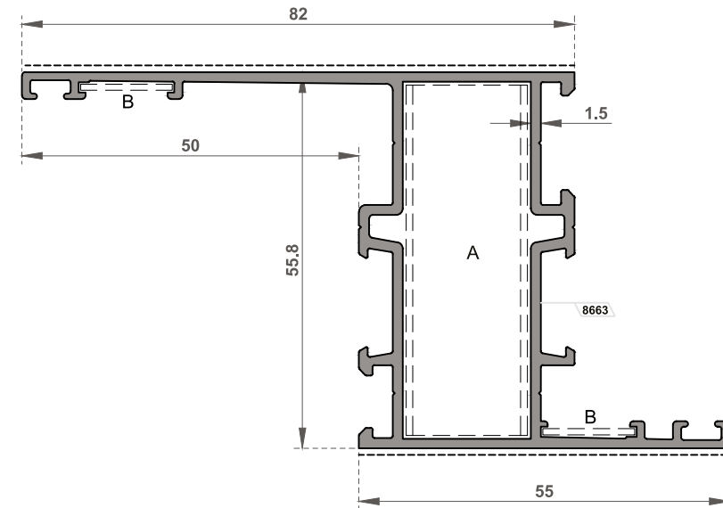
FI-1220 Kasa Profili 82/55 / Frame Profile 82/55 Et Kalınlığı / Wall Thickness 1.5mm
