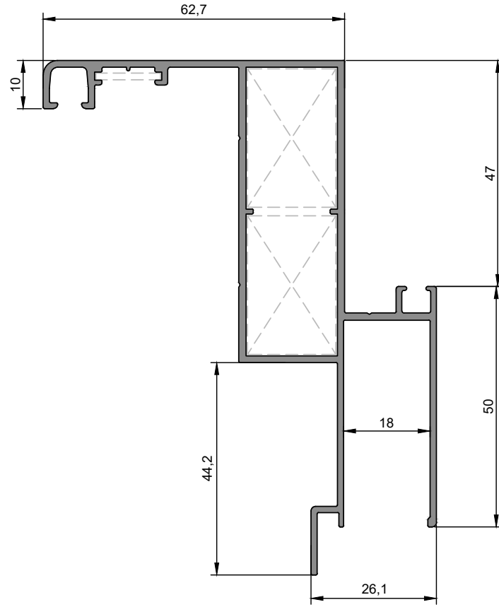
ER 9416 Kasa Profili / Frame Profile 1,366 kg/m
