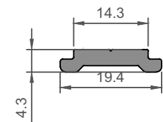
ER 8355 Tij Profili / Rod Profile Ağırlık / Weight 0,161 kg/m
