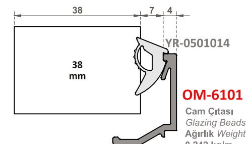
OM-6101 Cam Çıtası / Glazing Beads Ağırlık / Weight 0,242 kg/m
