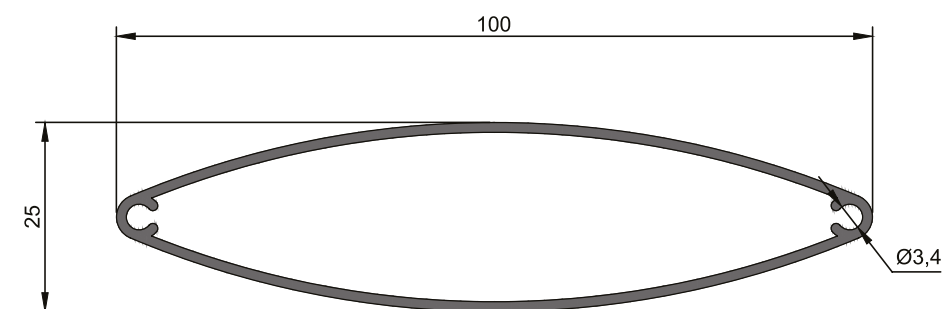
ER 6687 0,757 Kg/m
