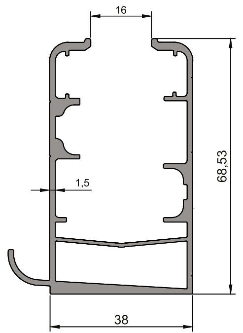
ER 6347 1,260 kg/m
