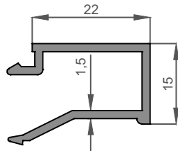
ER 3726 Çift Cam Çıtası Profili Glazing Bead Profile Ağırlık / Weight 0,286 kg/m
