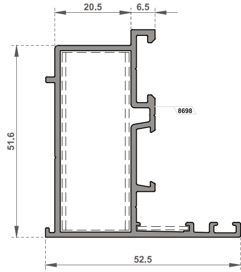
FI-5530 Dışa Açılır Adaptör Profili / Adapter Profile for Outwar Opening
