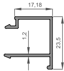
ER 6983 Cam Çıtası Profili Glazing Bead Profile Ağırlık / Weight 0,232 kg/m
