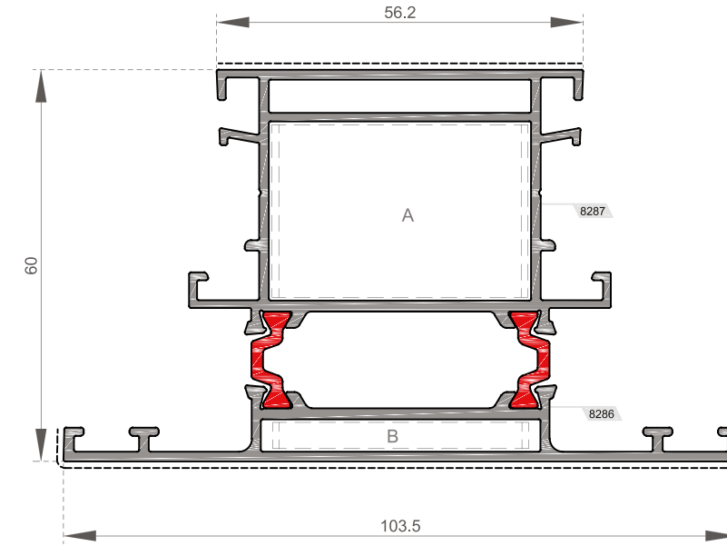
PS-2125 Geniş Orta Kayıt Profili 56.2 / 103.5 / Wide Mullion Profile 56.2 / 103.5 Et Kalınlığı / Wall Thickness 1.5mm
