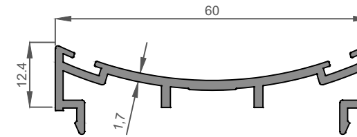
ER 3725 0,507 kg/m Çarpma Kapı Adaptör Profili Impact Door Adapter Profile
