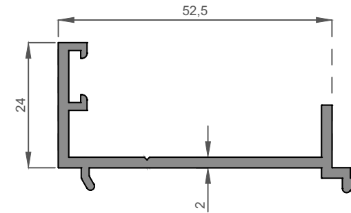
ER 3723 0,557 kg/m Kasa Adaptör Profili Case Adapter Profile
