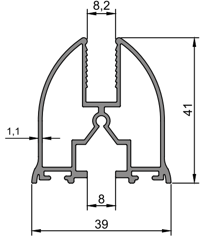
ER 7169 0,718 kg/m
