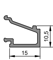
ER 9251 Cam Çıtası Profili Glazing Bead Profile 0,176 kg/m
