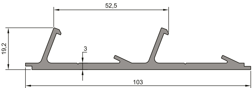
ER 9242 1,084 kg/m
