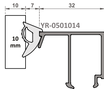
OM-6131 Cam Çıtası / Glazing Beads Ağırlık / Weight 0,351 kg/m
