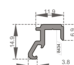
OM-5510 Etek Profili için Bağlantı Profili / Bottom Plate Adapter Profile Ağırlık / Weight 0,159 kg/m
