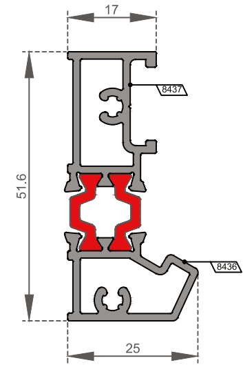
FS-5820 Alçak Eşik Profili / Low Threshold Profile Ağırlık / Weight 0,882 kg/m
