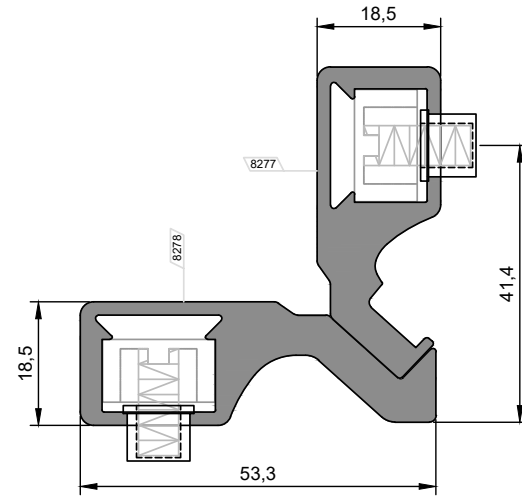
OM-5141 Yaylı Köşe Takoz Profili Springed Corner Cleat Profile 2,210 kg/m
