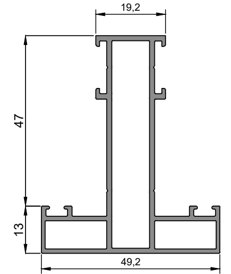
ER 9250 Orta Kayıt Profili Mullion Profile 0,919 kg/m
