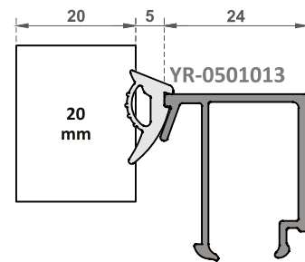
OM-6122 Cam Çıtası / Glazing Beads Ağırlık / Weight 0,318 kg/m
