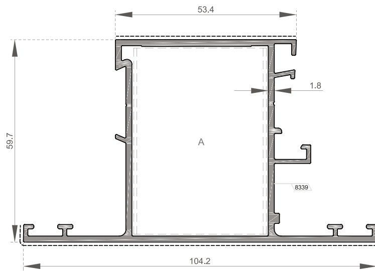
PA-1435 Geniş Orta Kayıttan Kasa Profili 53.4 / 104.2 / Wide T Frame Profile 53.4/ 104.2 Et Kalınlığı / Wall Thickness 1.8mm
