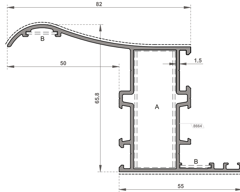
FI-1520 Kasa Profili 82/55 / Frame Profile 82/55 Et Kalınlığı / Wall Thickness 1.5mm
