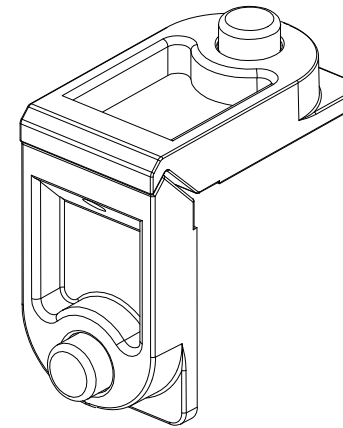
YR-0803005 KASA: Monticelli Köşe Takozu 0461/250 (L:29, H:18.4)
