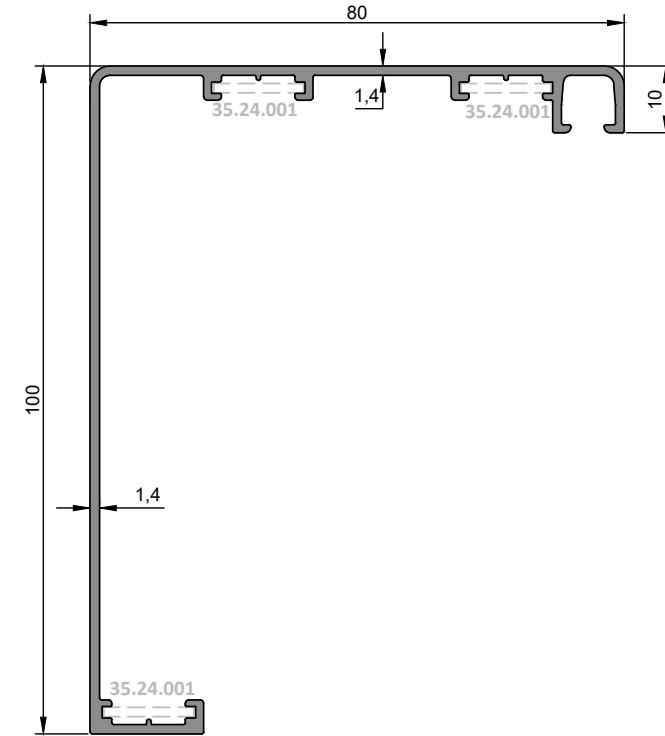
ER 9418 Pervaz 02 / Arcitrave Profile 02 0,908 kg/m
