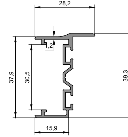
ER 9802 Orta Birleşim Adaptörü Mullion Adapter 0,374 kg/m
