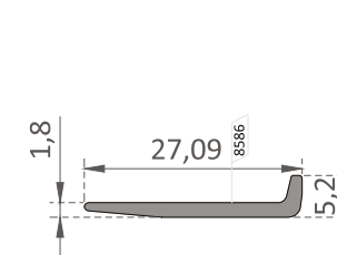
EL-2142 Cam Taşıyıcı Profili / Glass Support Profile
