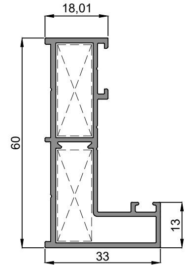
ER 9247 Kasa Profili Frame Profile 0,764 kg/m
