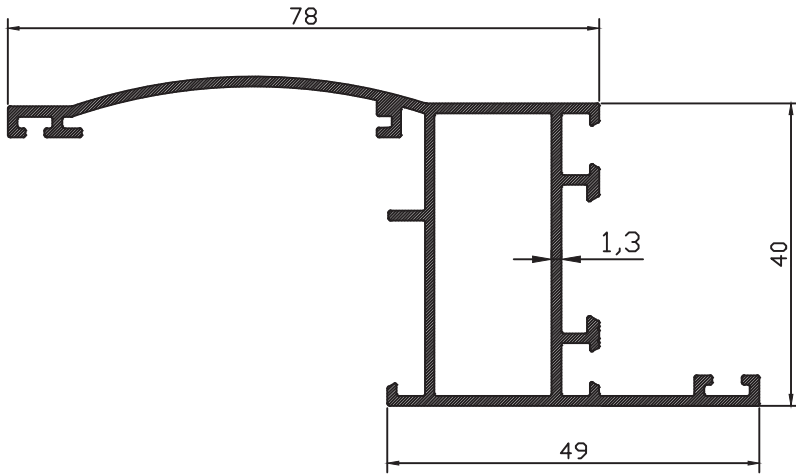
ER-7737 0,879 kg/m
