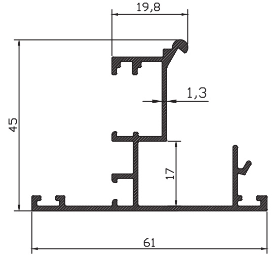
ER-7729 0,637 kg/m
