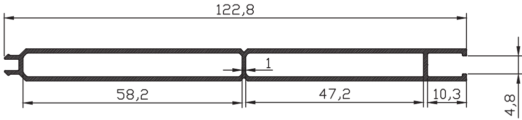
ER-7741 0,781 kg/m
