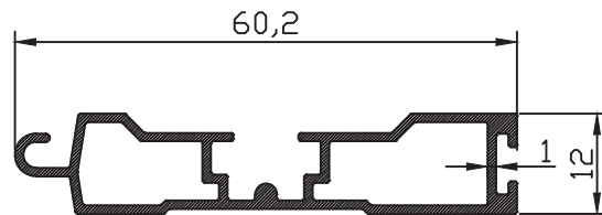
ER-7742 0,447 kg/m
