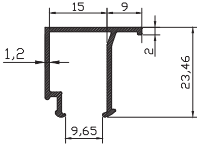
ER-7545 0,249 kg/m
