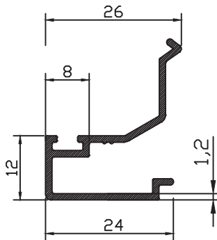
ER-7733 0,268 kg/m
