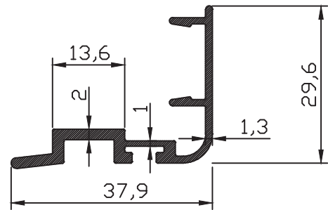
ER-7732 0,389 kg/m
