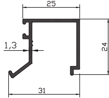
ER-7730 0,296 kg/m
