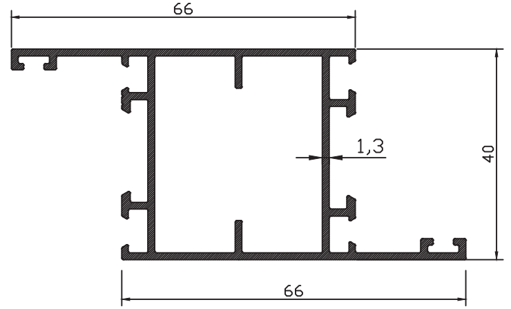
ER-7734 0,968 kg/m
