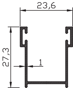
ER-7740 0,239 kg/m
