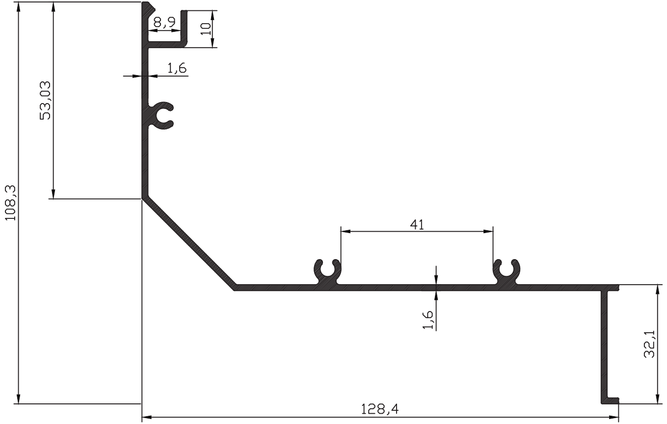
ER 7743 1,280 kg/m
