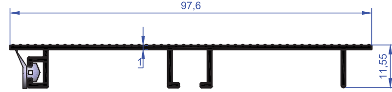
EMT - 840 BAZA FİTİLİ Base Gasget
