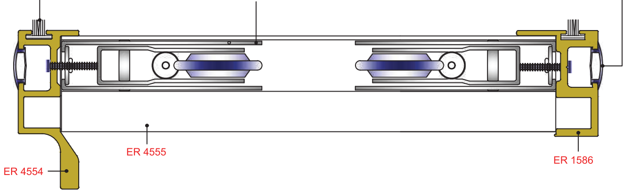
EMT - 820 67 / 700 SÜRME KAPAK KIL FİTİLİ Sliding Cover Brush Gasget
