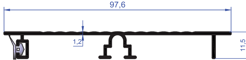
EMT - 840 BAZA FİTİLİ Base Gasget
