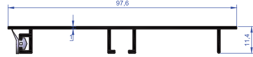
EMT - 840 BAZA FİTİLİ Base Gasget
