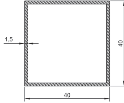
ER 4860 0,628 kg/m 40 X 40 X 1.5 Kutu Profili
