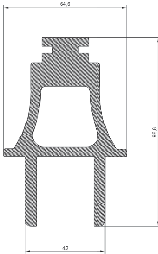
ER 4816 5,005 kg/m 60 LİK Dikma Mafsal Profili
