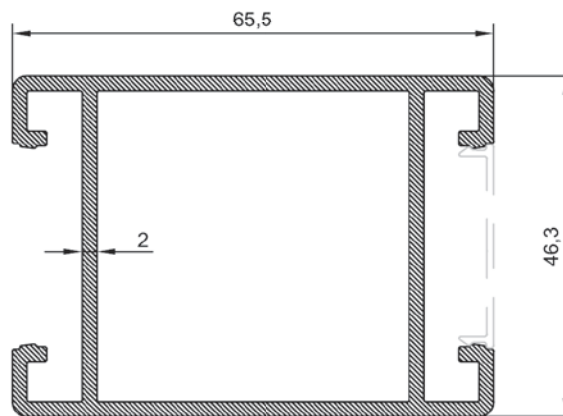
ER 4819 1,385 kg/m 40 X 60 Dikme Profili
