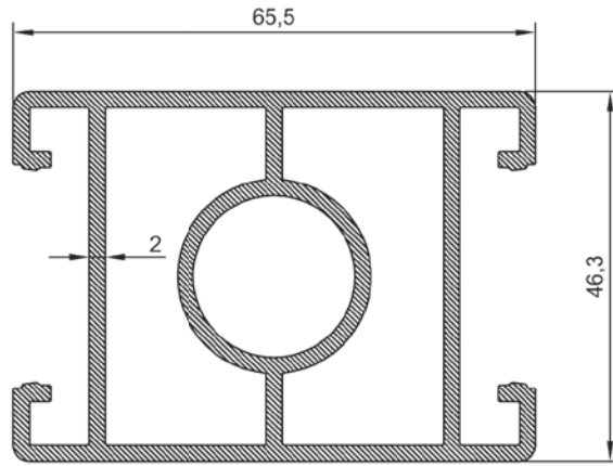
ER 4828 1,860 kg/m 40X60 Yuvarlak Ankrajlı Dikme
