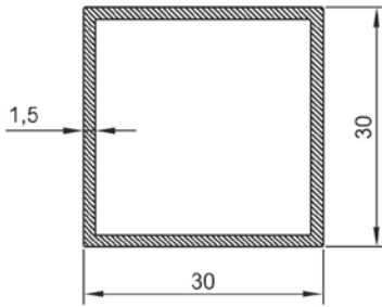
ER 4853 0,464 kg/m 30 X 30 X 1.5 Kutu Profili
