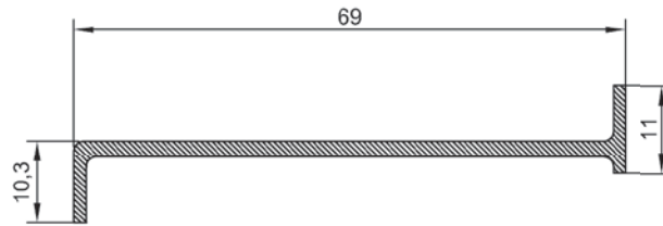
ER 4854 0,448 kg/m 69 X 15 X 2 Cam Yataklama Profili
