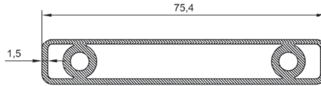
ER 4856 0,923 kg/m 40 X 80 ve 30x80 Duvar Ankrājı
