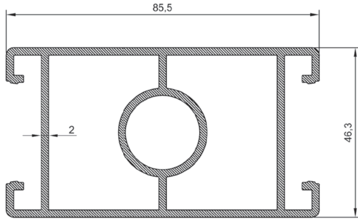
ER 4827 2,080 kg/m 40X80 Yuvarlak Ankrajlı Dikme
