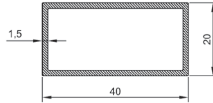
ER 4861 0,467 kg/m 20 X 40 X 1.5 Kutu Profili
