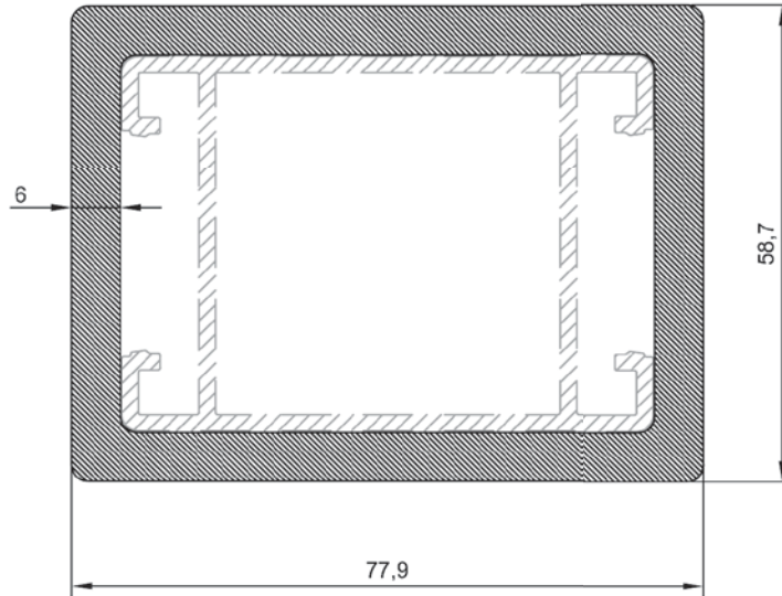
ER 4857 4,051 kg/m 40 X 60 Dikma Flanşı
