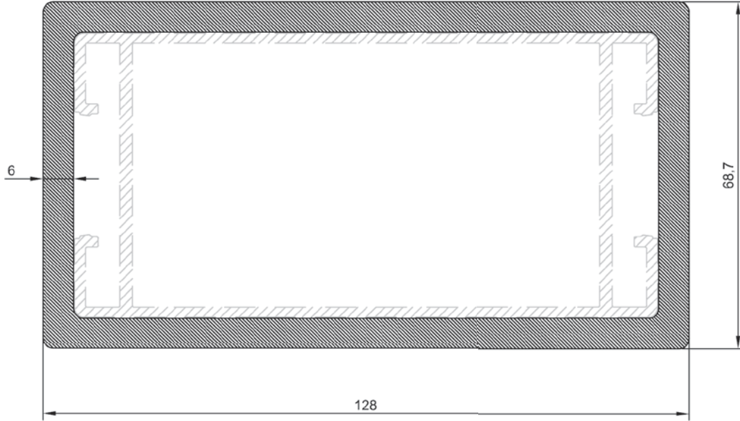
ER 4855 6,005 kg/m 50 X 120 Dikma Flanşı
