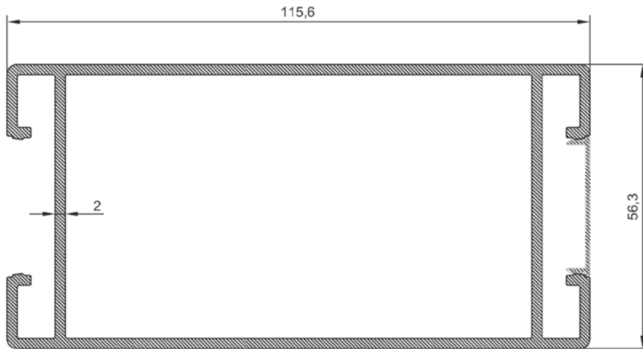
ER 4817 2,145 kg/m 50 X 120 Dikme Profili
