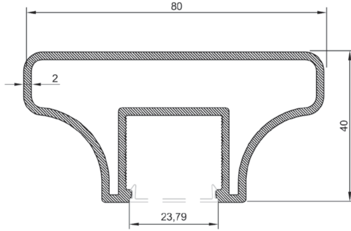
ER 4822 1,394 kg/m 40 X 80 Küpeşte Profili
