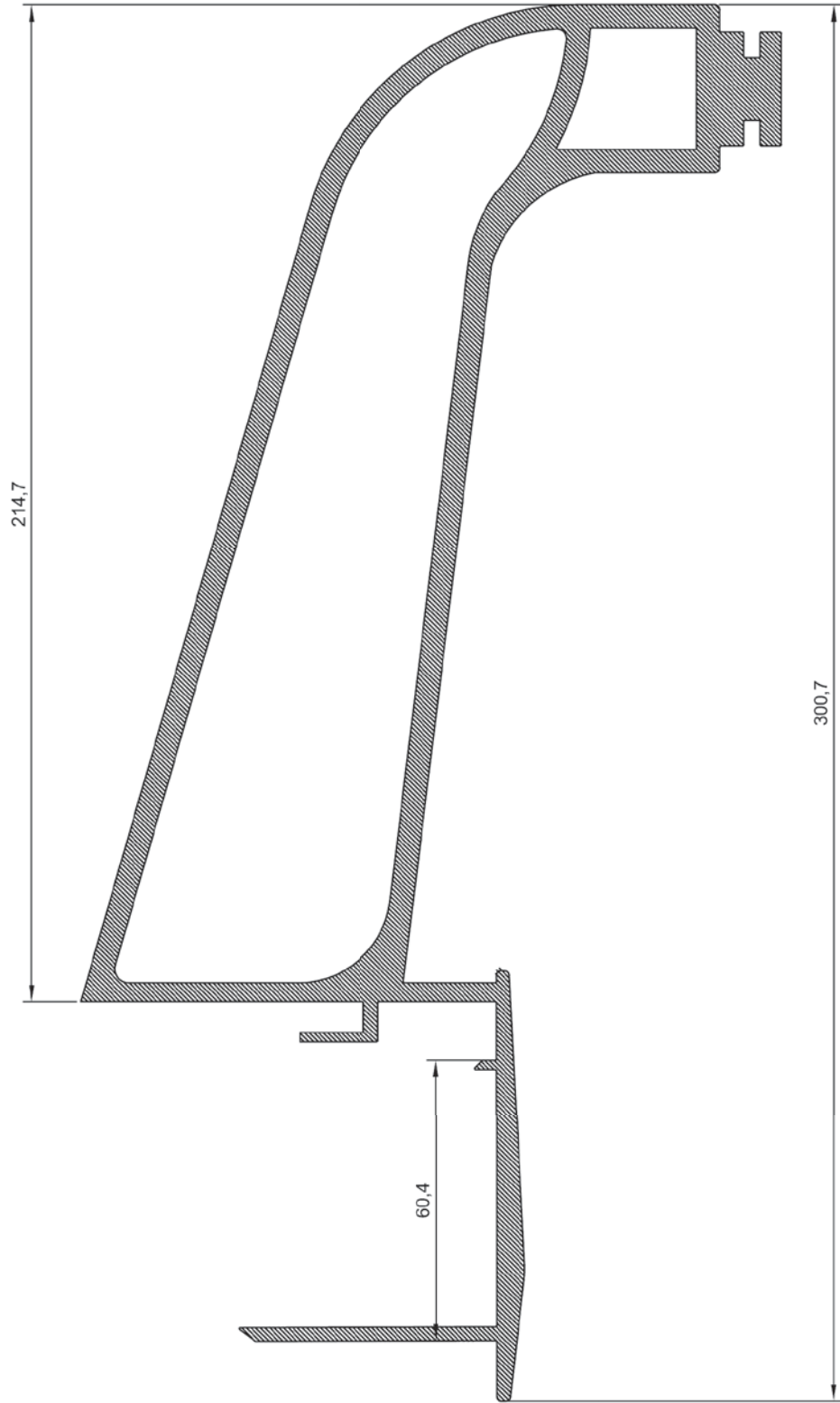
ER 4831 11,282 Kg/m 20cm.Kapaklı Mafsal Profili
