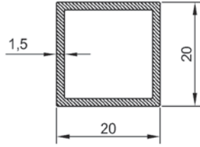
ER 4852 0,300 kg/m 20 X 20 X 1.5 Kutu Profili
