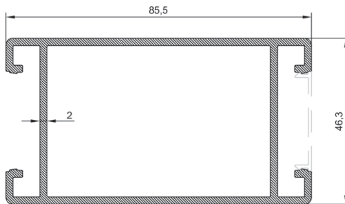
ER 4818 1,600 kg/m 40 X 80 Dikme Profili
