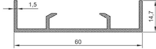
ER 4851 0,427 kg/m Ankrāj Gizleme Kapak Profili
