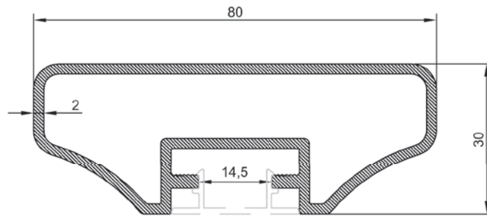
ER 4823 1,247 kg/m 30 X 80 Küpeşte Pprofili
