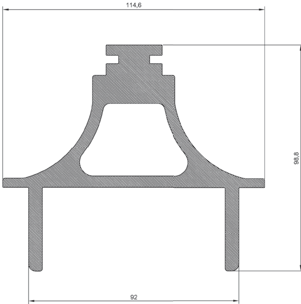
ER 4814 5,989 kg/m 120 LİK Dikma Mafsal Profili
