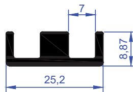
ER 5955 0,344 kg/m
