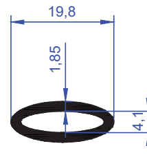
ER 6010 0,188 kg/m
