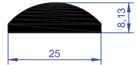
ER 6091 0,432 kg/m
