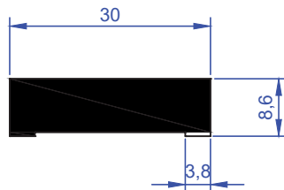
ER 5693 0,662 kg/m
