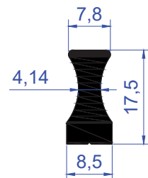
ER 6183 0,296 Kg/m
