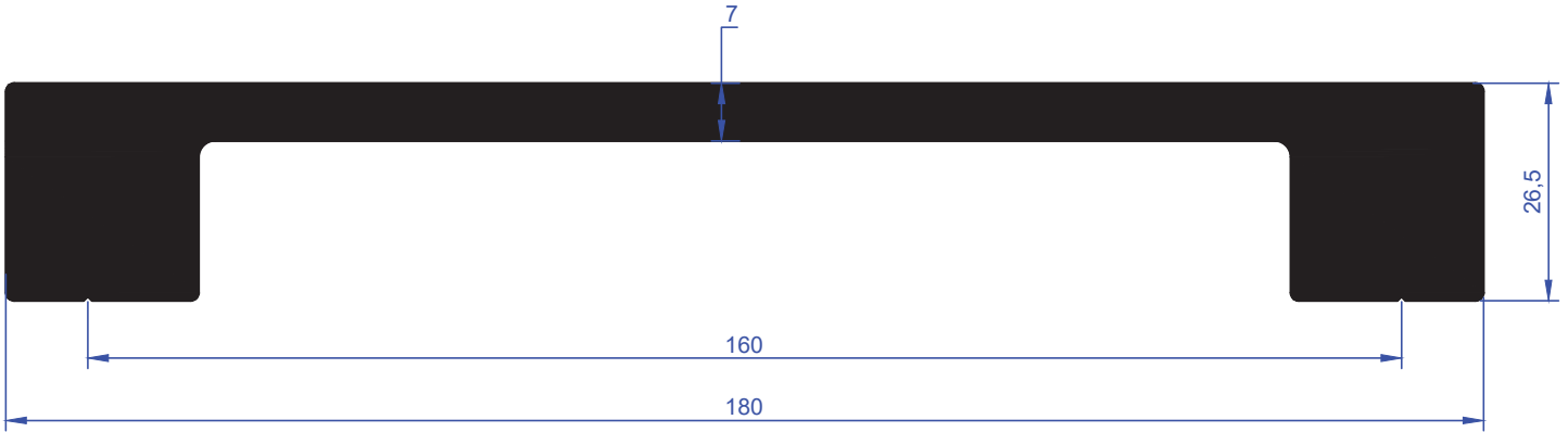
ER 2065 5,865 kg/m
