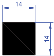
ER 5423 0,531 Kg/m
