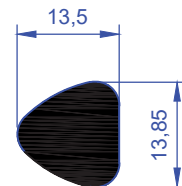
ER 6471 0,384 Kg/m
