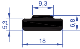
ER 4259 0,292 kg/m
