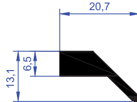
ER 6058 0,257 kg/m
