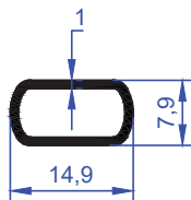
ER 4902 0,101 kg/m
