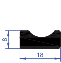
ER 5009 0,322 kg/m
