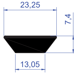
ER 6329 0,374 Kg/m
