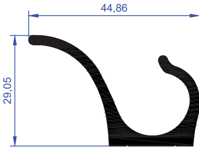
ER 5633 2,639 kg/m
