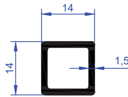
ER 5884 0,203 kg/m
