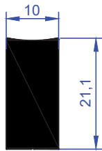
ER 5883 0,564 kg/m
