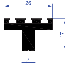
ER 5688 0,551 kg/m
