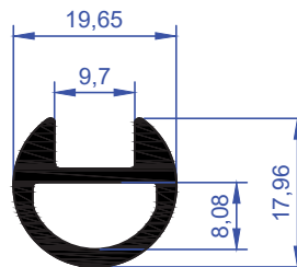
ER 5966 0,357 kg/m
