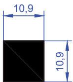
ER 5421 0,322 Kg/m
