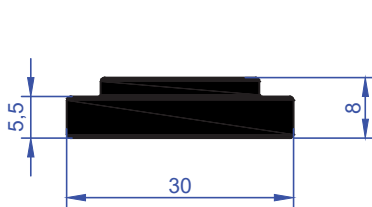
ER 6167 0,588 kg/m
