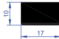
ER 1493 0,479 kg/m
