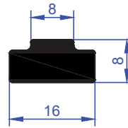
ER 4801 0,314 kg/m
