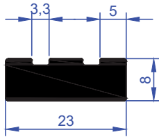
ER 4896 0,477 kg/m
