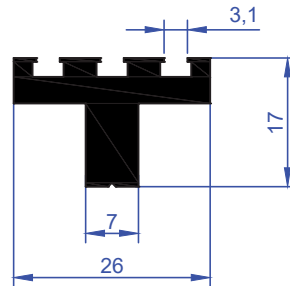
ER 5688 0,551 kg/m
