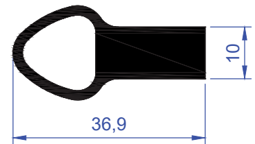
ER 6469 0,773 Kg/m
